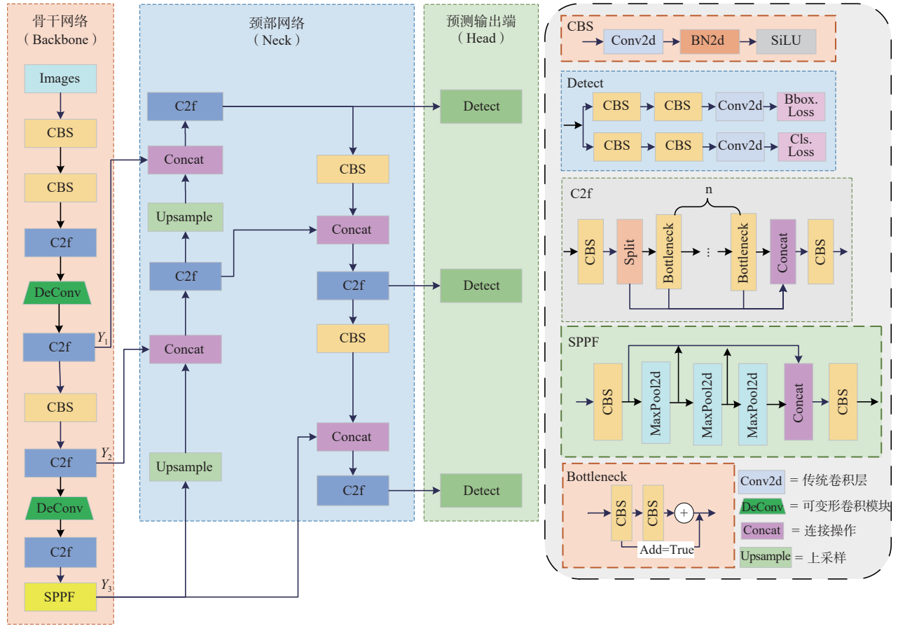
图1 基于可变形卷积的安全帽佩戴检测框架
