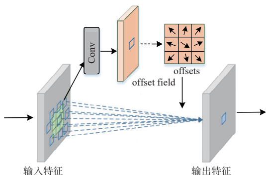
图2 可变形卷积模块
