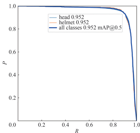
图6 本文模型的精确率-召回率曲线
