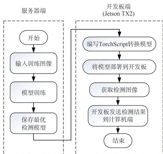
图8 基于嵌入式开发板的目标检测系统流程
